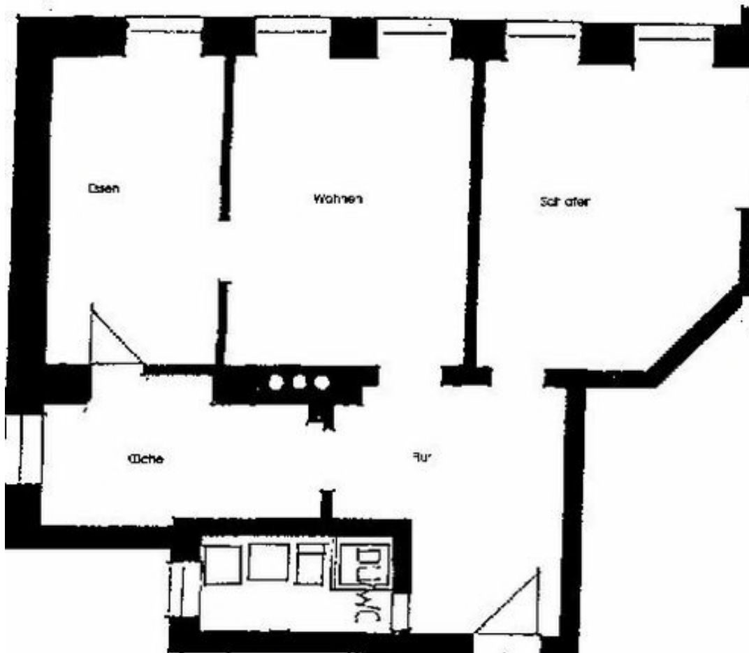
Grundriss
