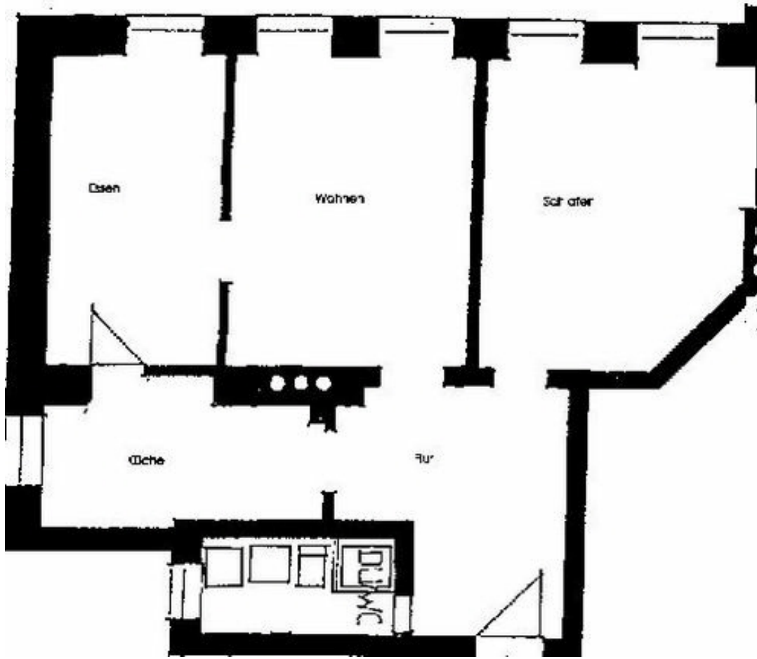
Grundriss
